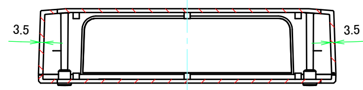
B-B ( 1 : 3 )
